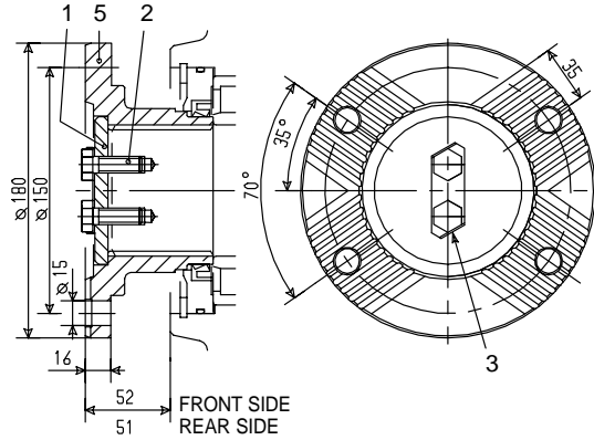
KIT 2.05.389.0000 180 ISO 8667
