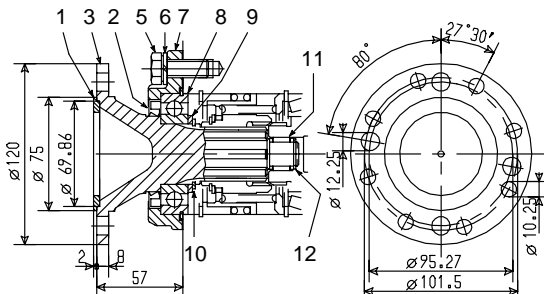
KIT 2.05.349.0000 SPICER 1410 / DIN 20
